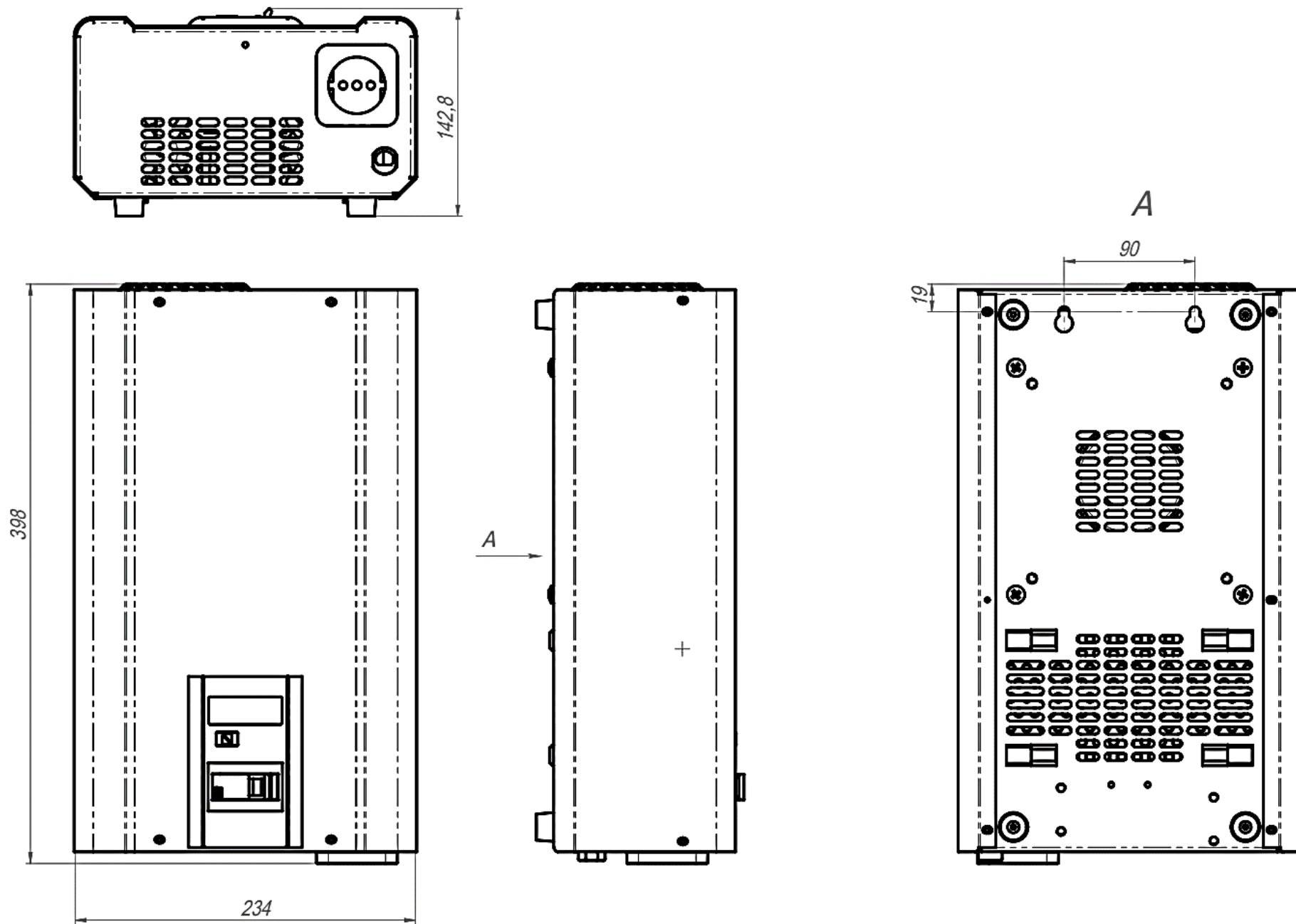
Габаритные и установочные размеры стабилизаторов АМПЕР на 10 и 16А
