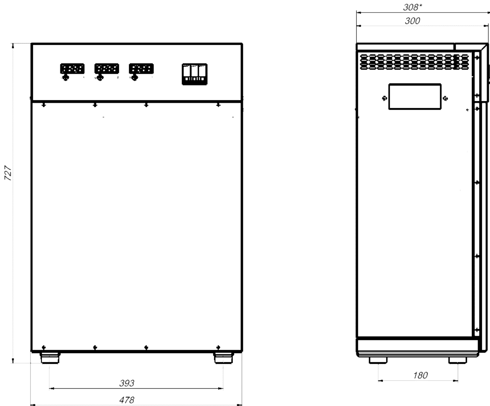
Габаритные размеры стабилизаторов Ампер на 25-63А
