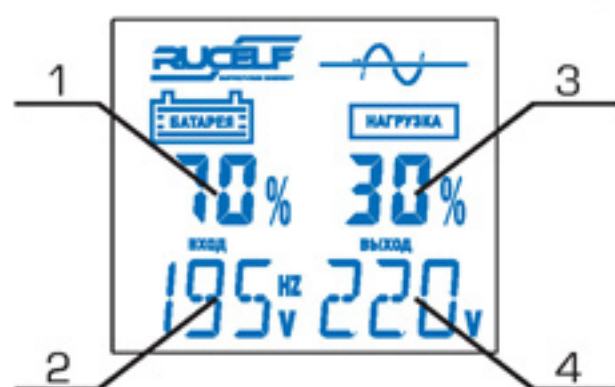
Рис. 1 Дисплей ИБП
