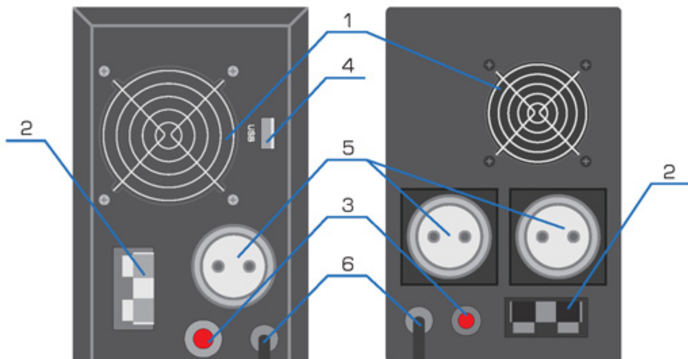
Рис. 3 Задняя панель ИБП
