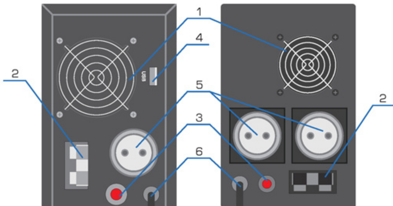
Рис. 3 Задня панель ДБЖ
