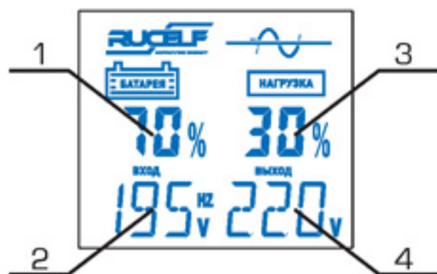
Рис. 1 Дисплей ДБЖ
