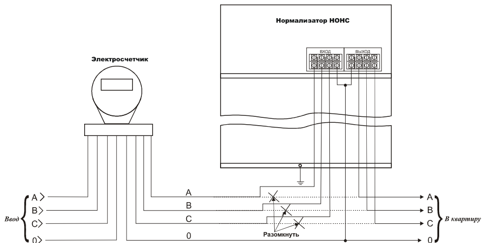
Рисунок 5. Подключение нормализатора.
