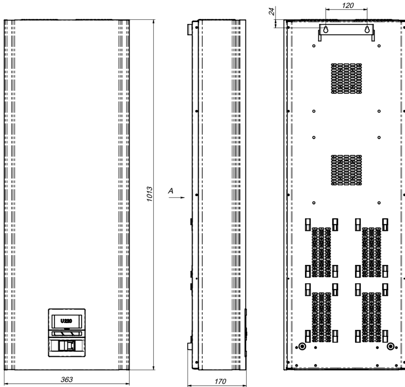
Установочные и посадочные размеры стабилизаторов Герц и на 100-125 А
